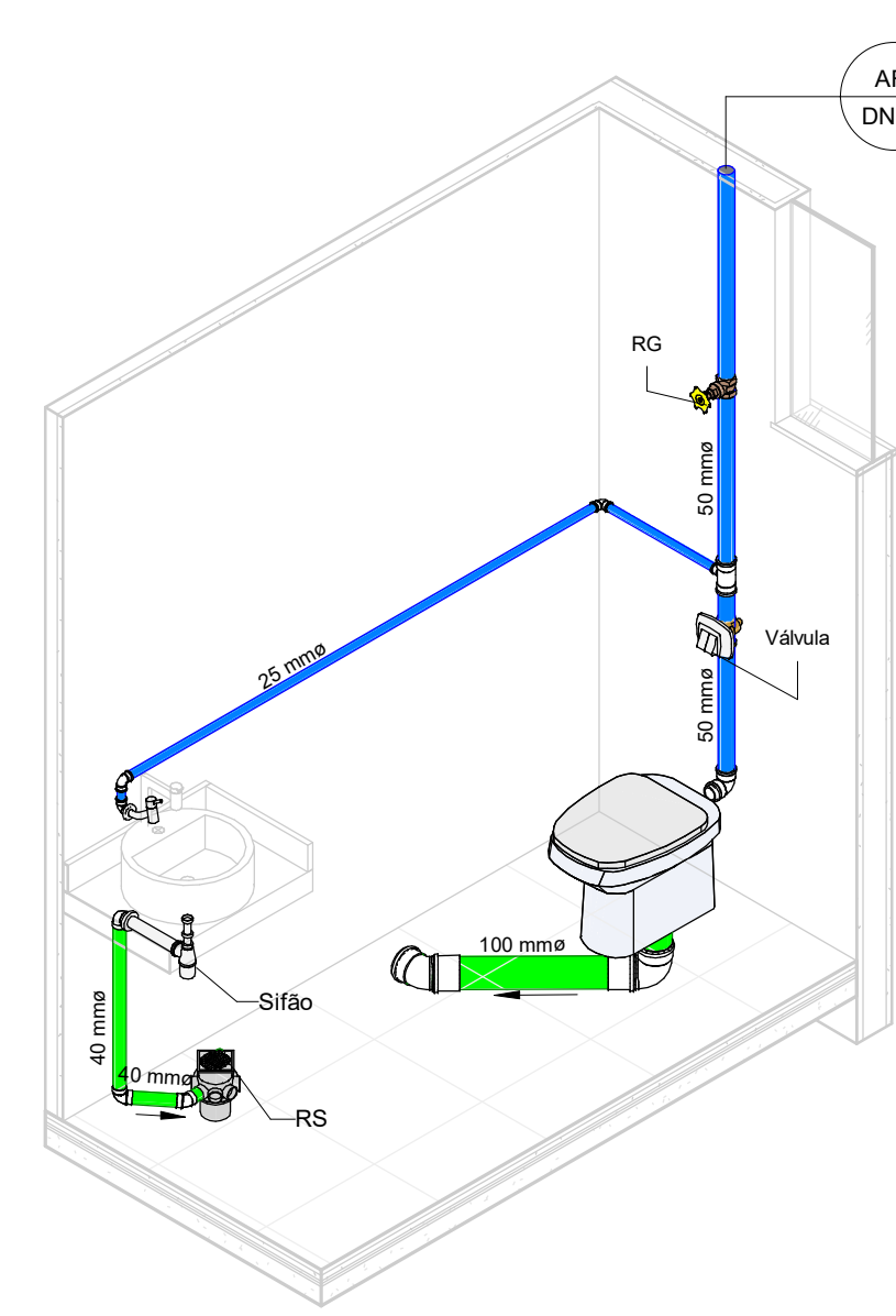
6 ISOMÉTRICO BH2
