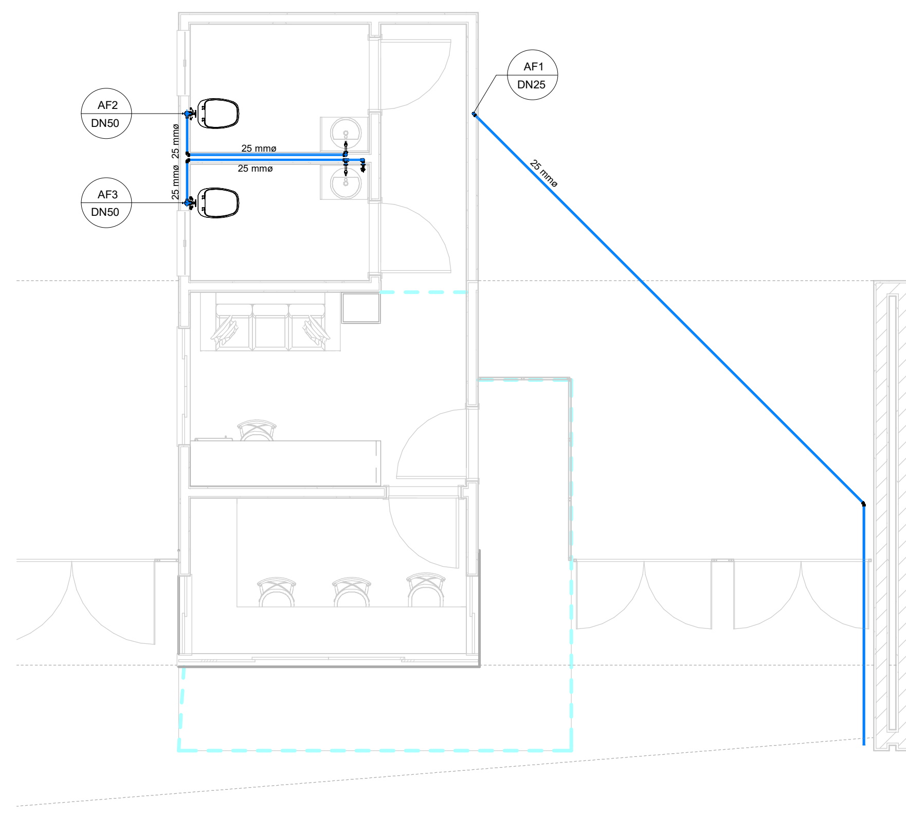
2 AF - Nível 1 1 : 50
