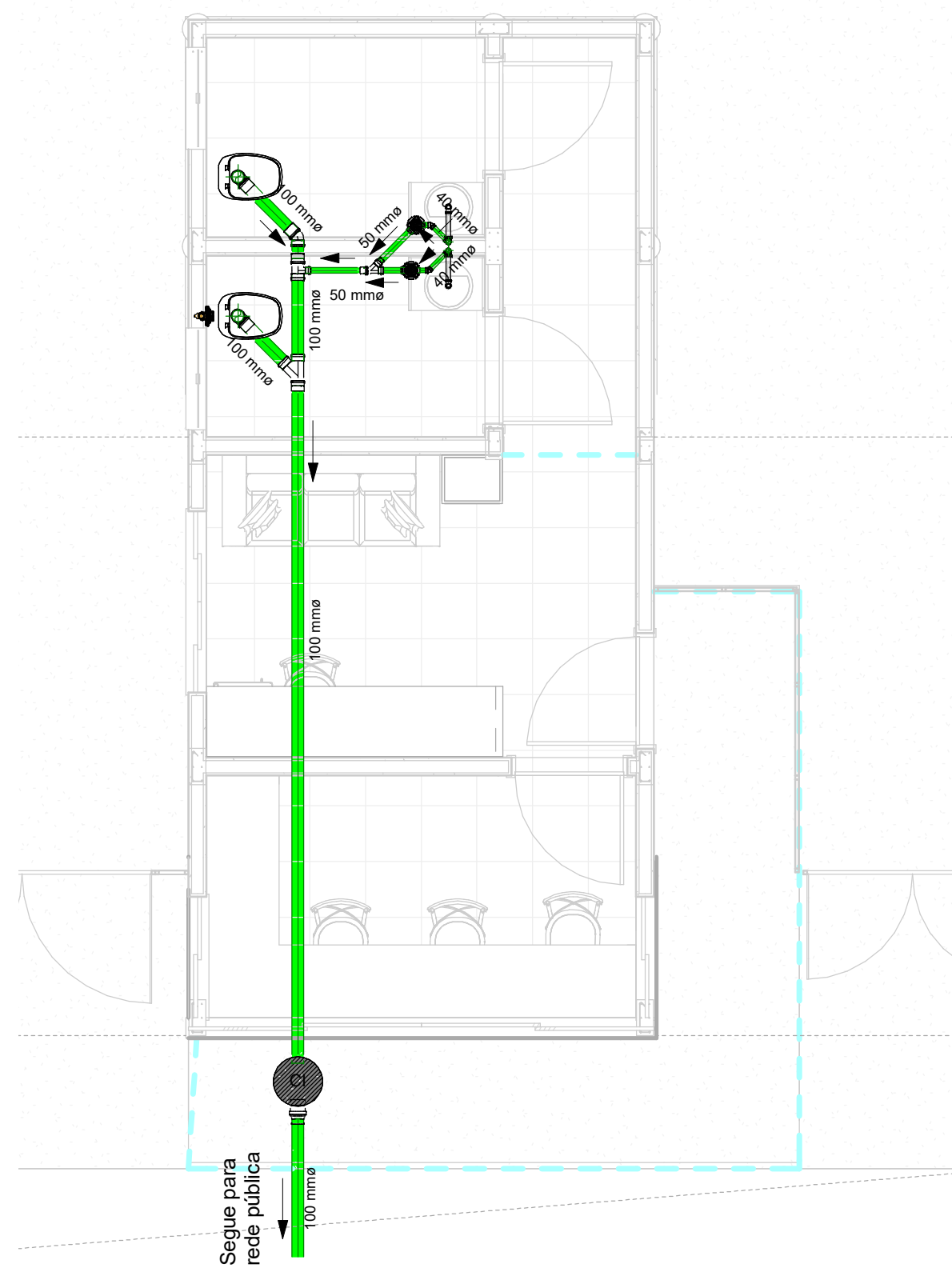
1 ESG - Nível 1 1 : 50
