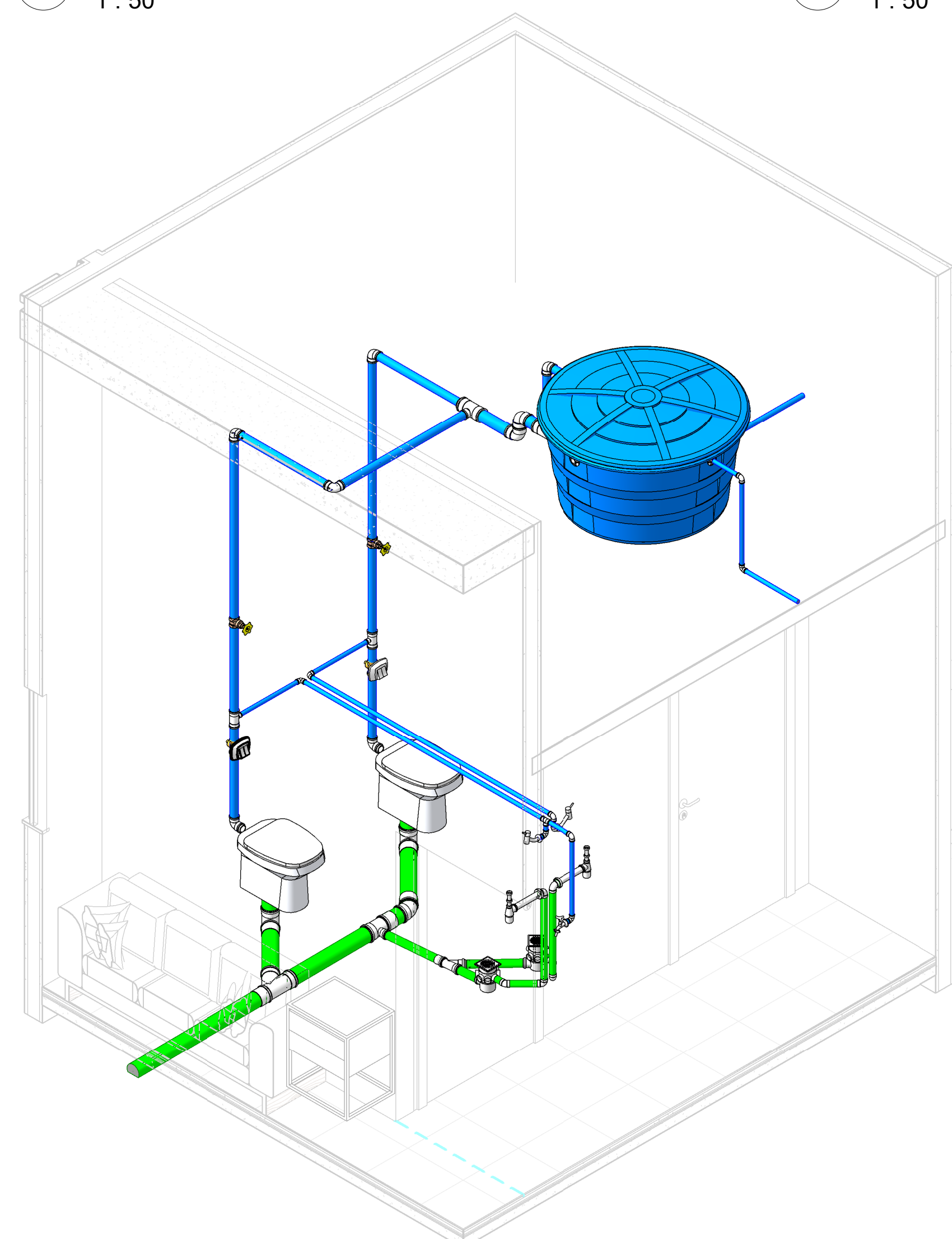
4 GERAL - ISOMÉTRICO
