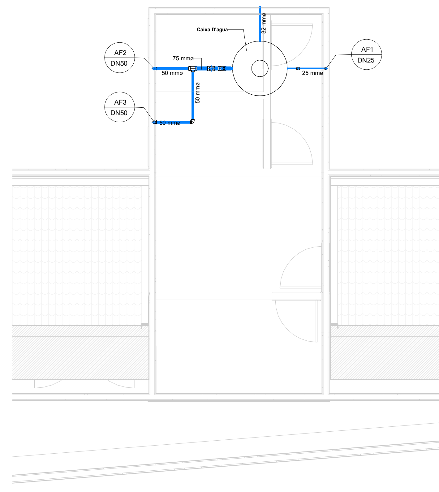
3 AF - Nível 2 1 : 50
