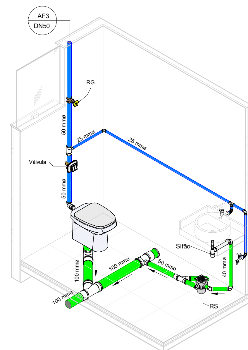
5 ISOMÉTRICO BH1
