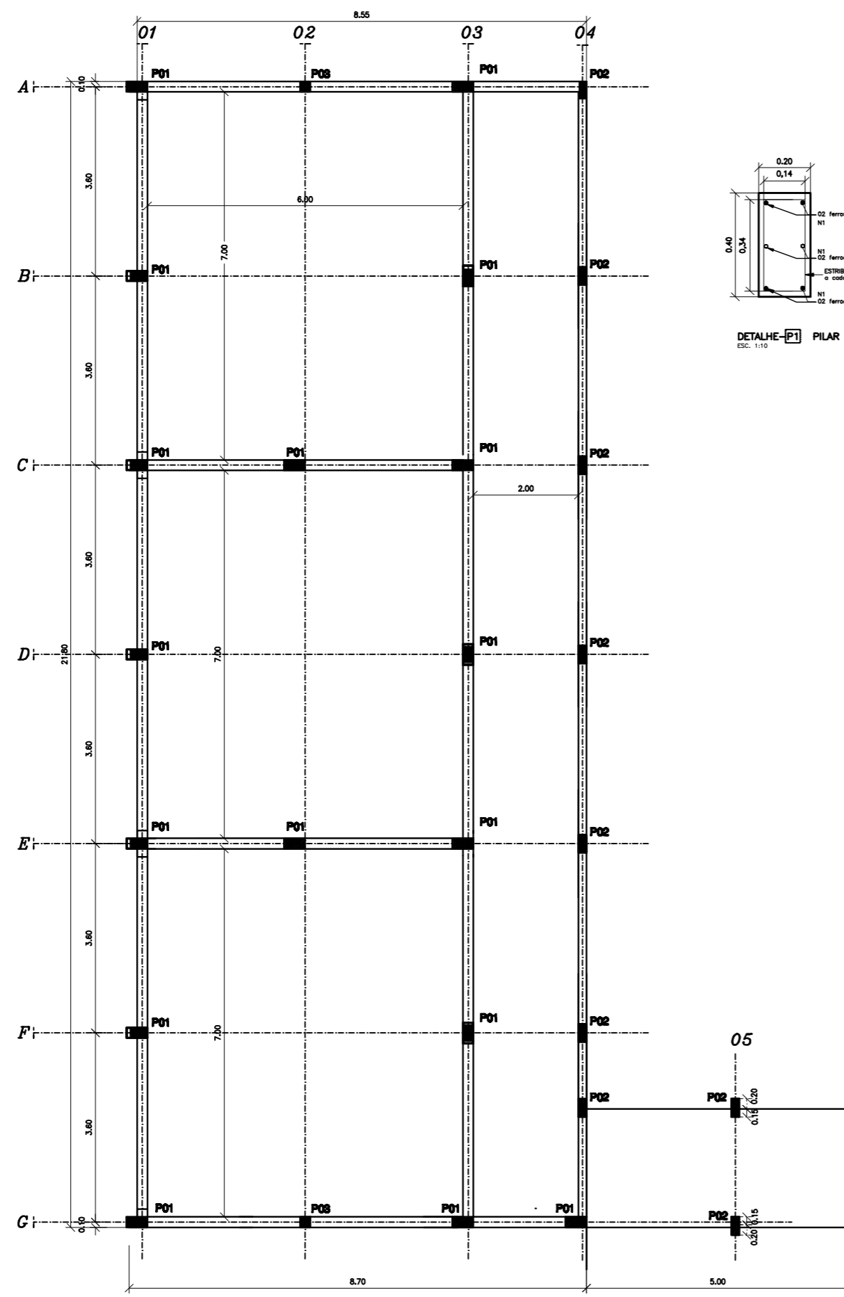
PLANTA BAIXA- FUNDAÇÃO PONTOS DE BROCAS/FILARES ESC. 1:50
