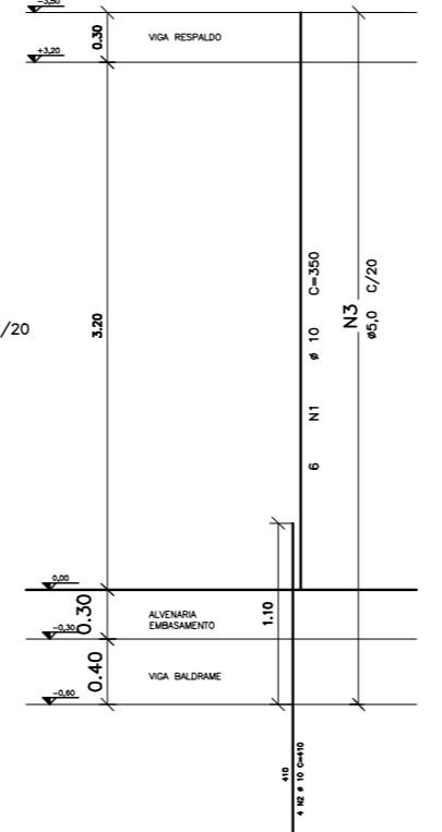
FORMA DETALHE-P1 20x40 (17)
