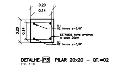
FORMA DETALHE-P3 20x20 (02)
