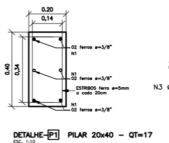
DETALHE-P1 PILAR 20x40 - QT=17 ESC. 1:10
