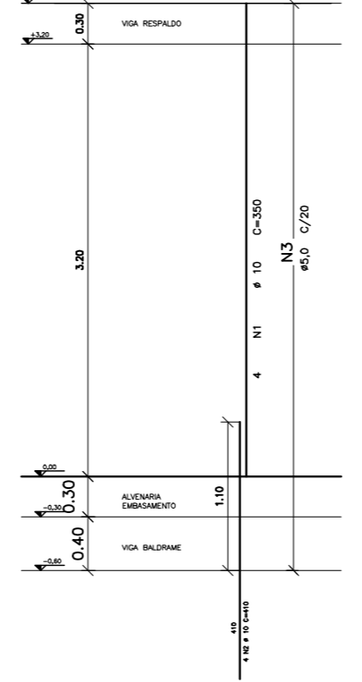
FORMA DETALHE-P3 20x20 (02)
