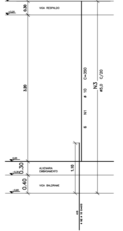
FORMA DETALHE-P2 15x35 (09)
