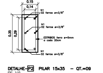
DETALHE-P2 PILAR 15x35 - QT=09 ESC. 1:10
