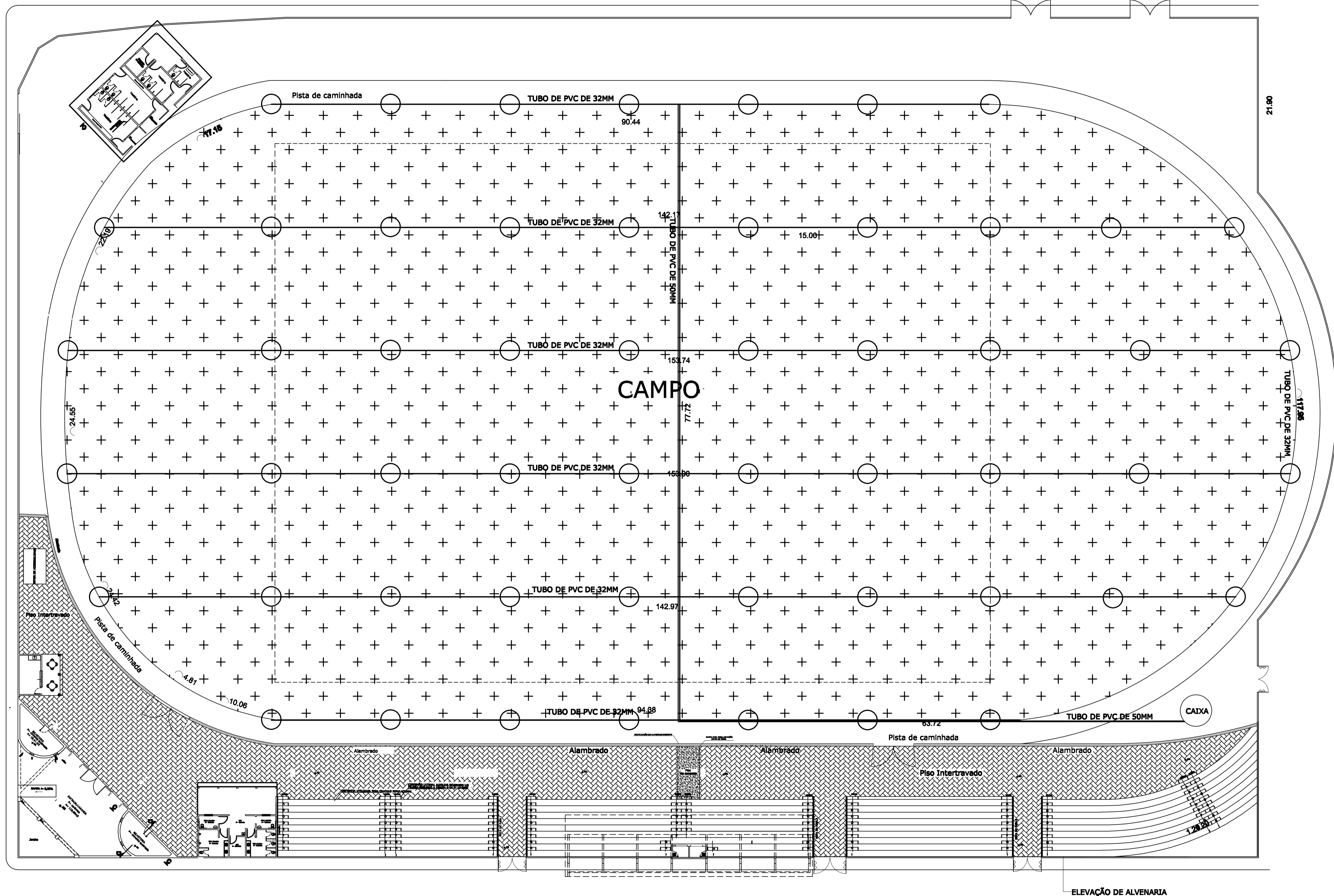
SITUAÇÃO PRETENDIDA 1:200
