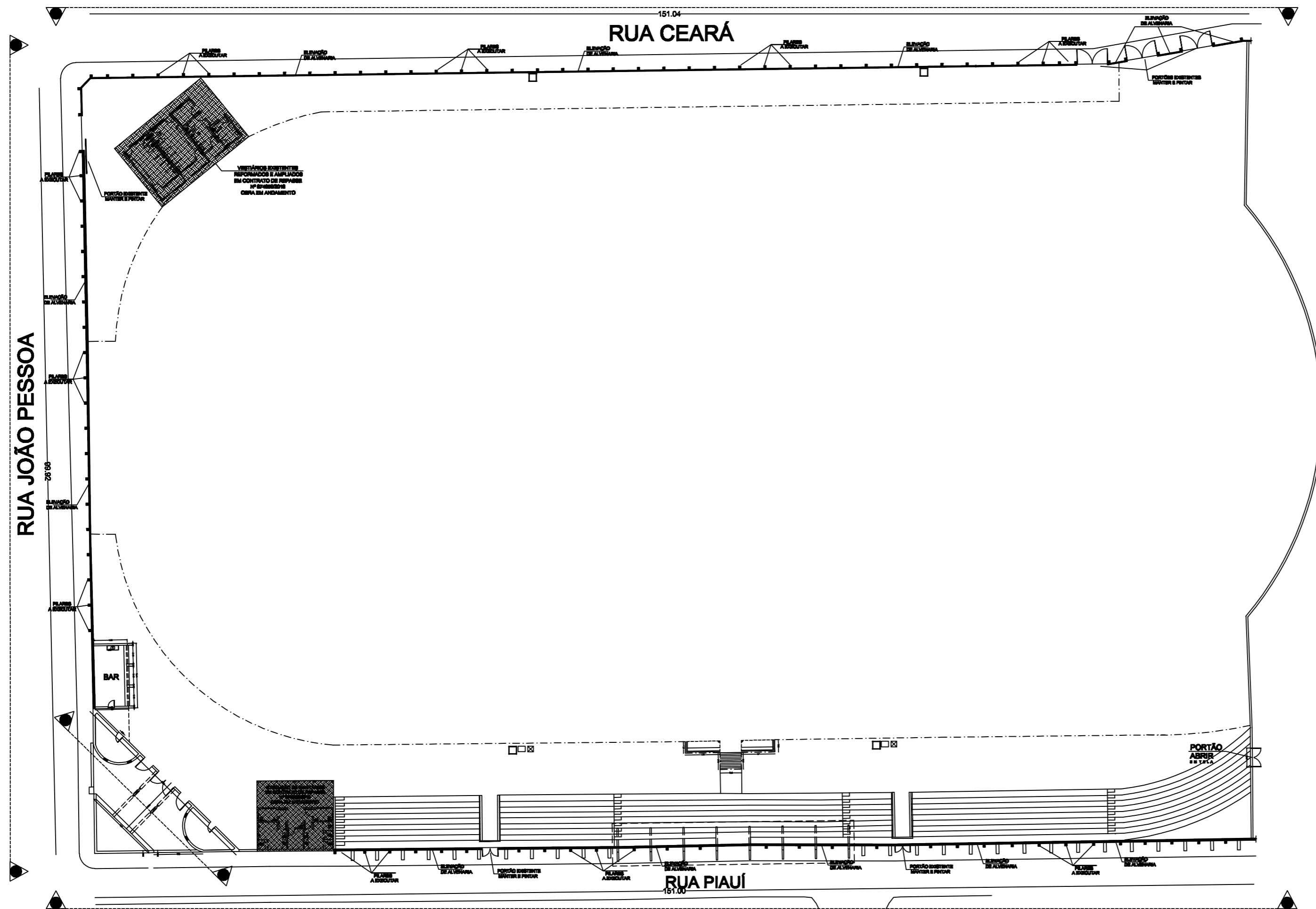
PLANTA SERVIÇOS A EXECUTAR 1:300
