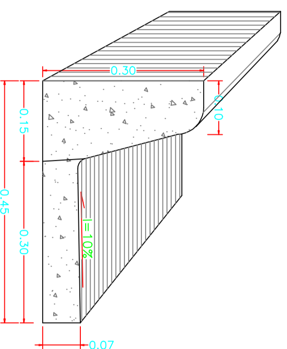
DET. A - GUIA E SARJETA EESC 1:1.000 Obs.: Guias e Sarjetas serão executadas extruzidas "in loco"
