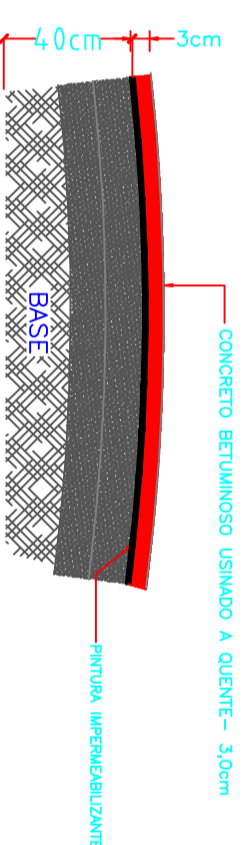
DET. REVESTIMENTOS s/ EESC
